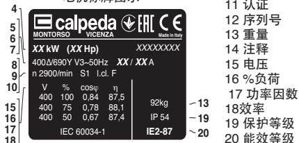
电机标牌图示
