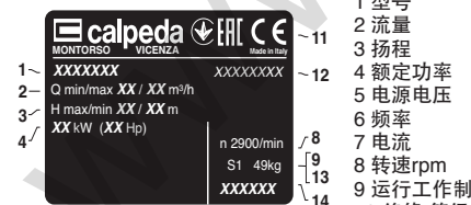
电机标牌图示
