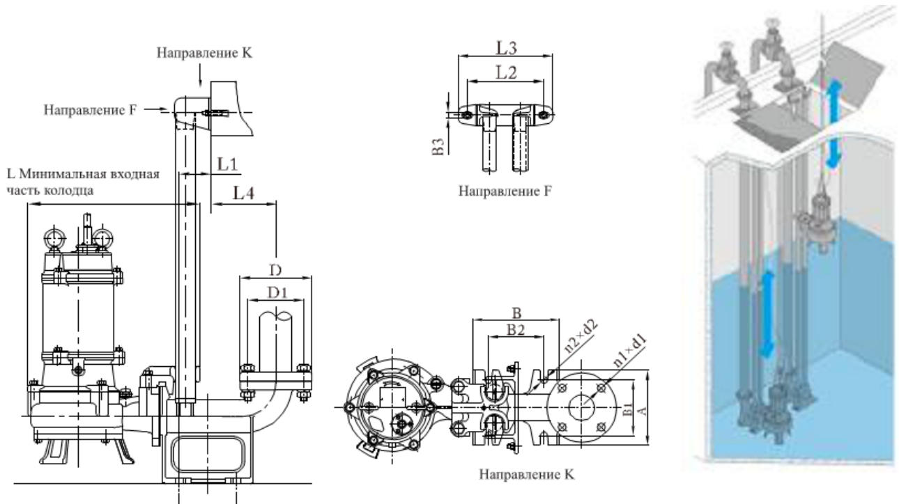
Рис. 5 Стационарная установка насосов WQ/WQS/WQQG/WQA/WQAS/WQV/KBD/KBS/L при помощи автоматической трубной муфты
