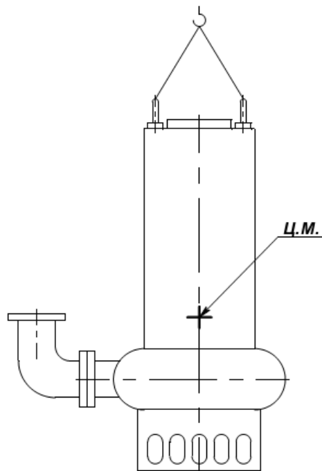
Рис. 2 Схема строповки насоса без тары
