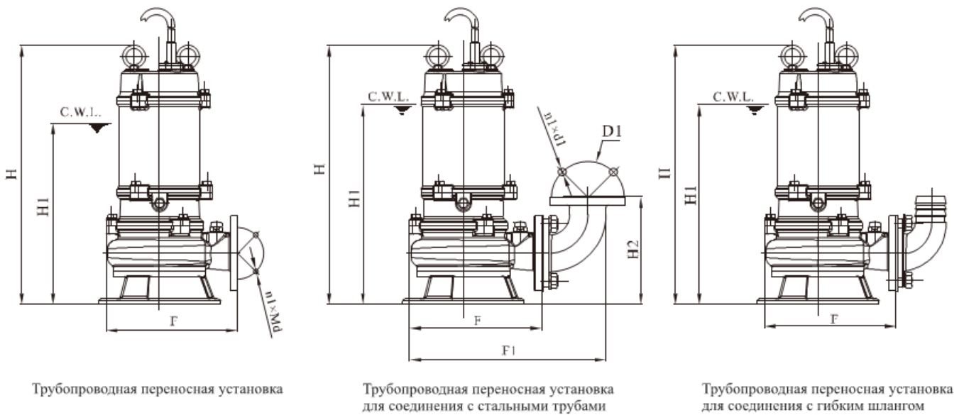
Рис. 6 Переносная установка насосов WQ/WQS/WQQG/WQA/WQAS/WQV/KBD/KBS/L
