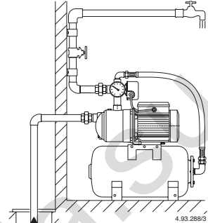
Fig. 2 Funzionamento in aspirazione Suction lift operation Saugbetrieb Fonctionnement en aspiration Funcionamiento en aspiración Sugande funktion Zuigsituatie Θέση λειτουργίας με κάθστη αναρρόφηση Работа выше уровня жидкости 负压水头工作
