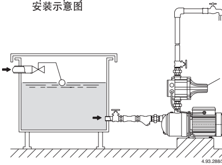
Fig. 1 Funzionamento sotto battente Positive suction head operation Zulaufbetrieb Fonctionnement en charge Funcionamiento bajo carga Tillrinning sugsidan Toelooptituatie Θέση λειτουργίας με θετική αναρρόφηση Работа под гидравлическим напором 正吸上水头的操作
